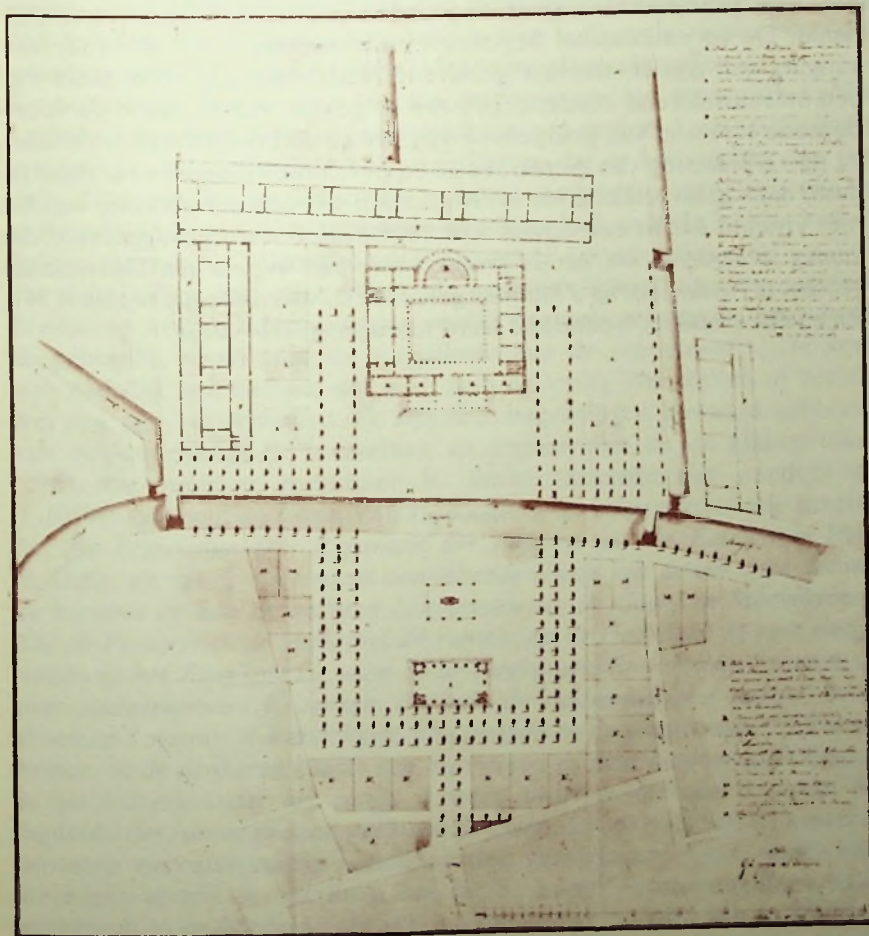
Het andere plan van Giudici: Già presso al termine; dit idee werd het uitgangspunt van de commissie voor verdere ontwerpen. Algemeen Rijksarchief, Den Haag.
