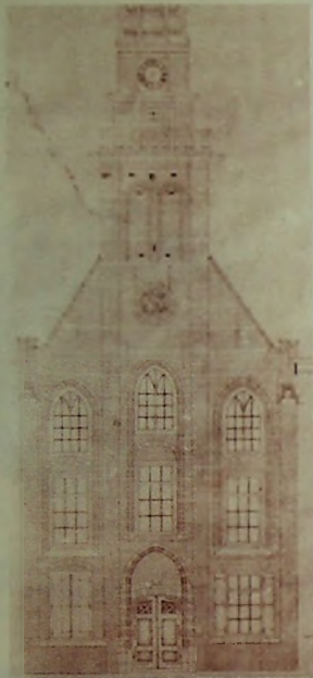
De laatgotische voorgevel van de Sint Jacobskapel, bij de opmeting vóór de restauratie in 1956.
