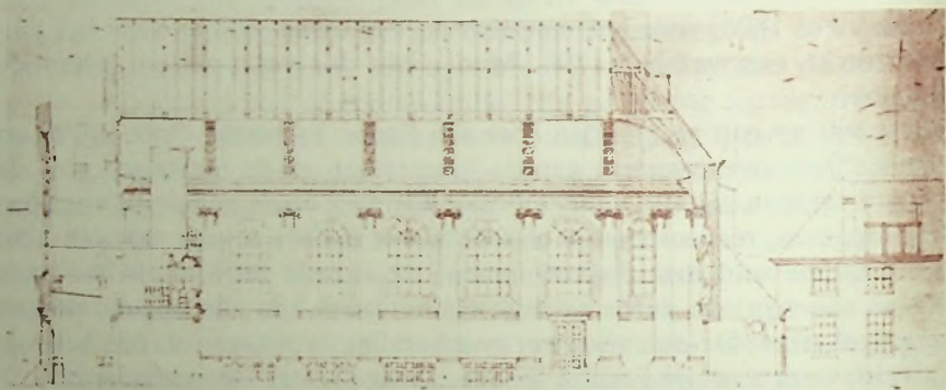
Doorsnede van de Lodewijkskerk; opmetingstekening vóór de restauratie en verbouwing van 1956. Lodewijksarchief.
